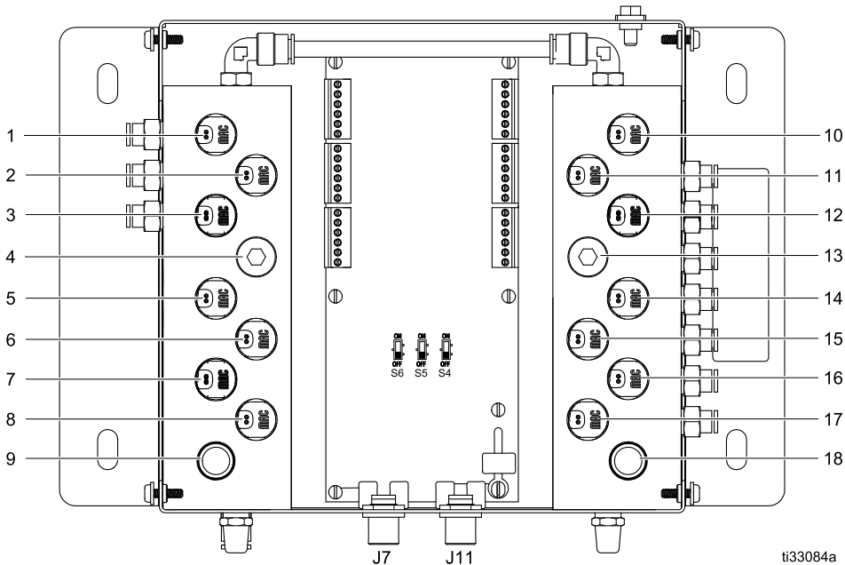
Figure 55 솔레노이드 위치 일람표
