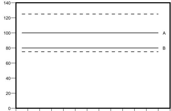
Figure 46 목표 스프레이 압력(A)이 100psi이고 혼합 압력 공차가 25%인 시스템의 허용 가능한 B 쪽 펌프 배출구 압력 범위
