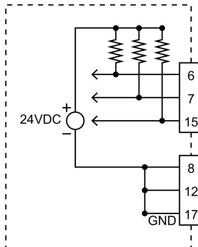
Figure 2 Digitale uitgangen - Sinking-uitgangen met externe "pull-up" weergegeven
