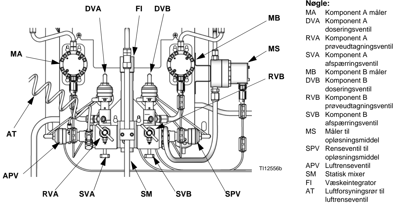
Fig. 67. Vægmonteret væskestation
