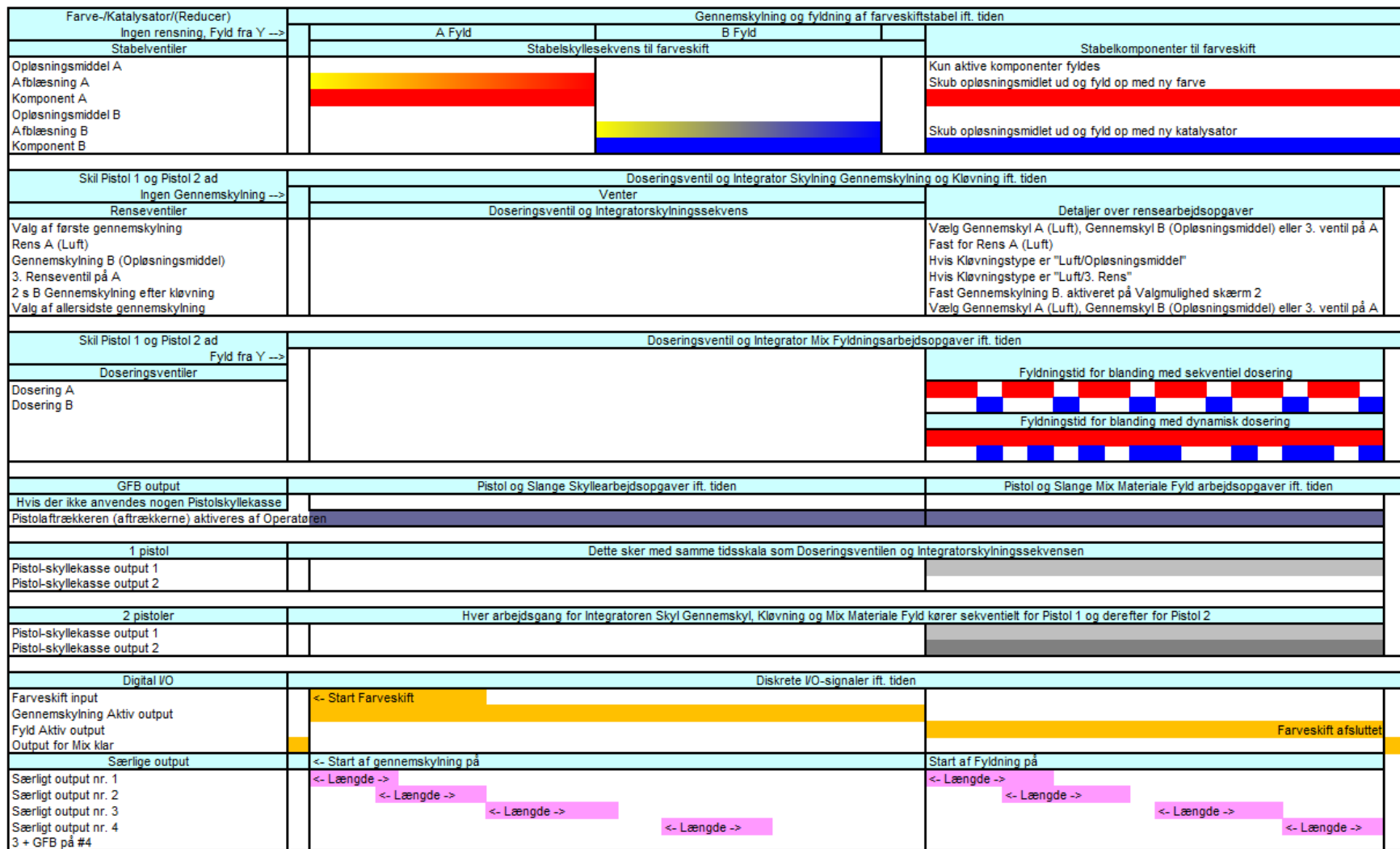
ProMix 2KS Diagram over opskriftfyldning nr. 4 0 til Y Stabelventiler A1, B1 Afbløsning A aktiveret, 3. Skyllventil aktiveret Ingen udgående fyldning
