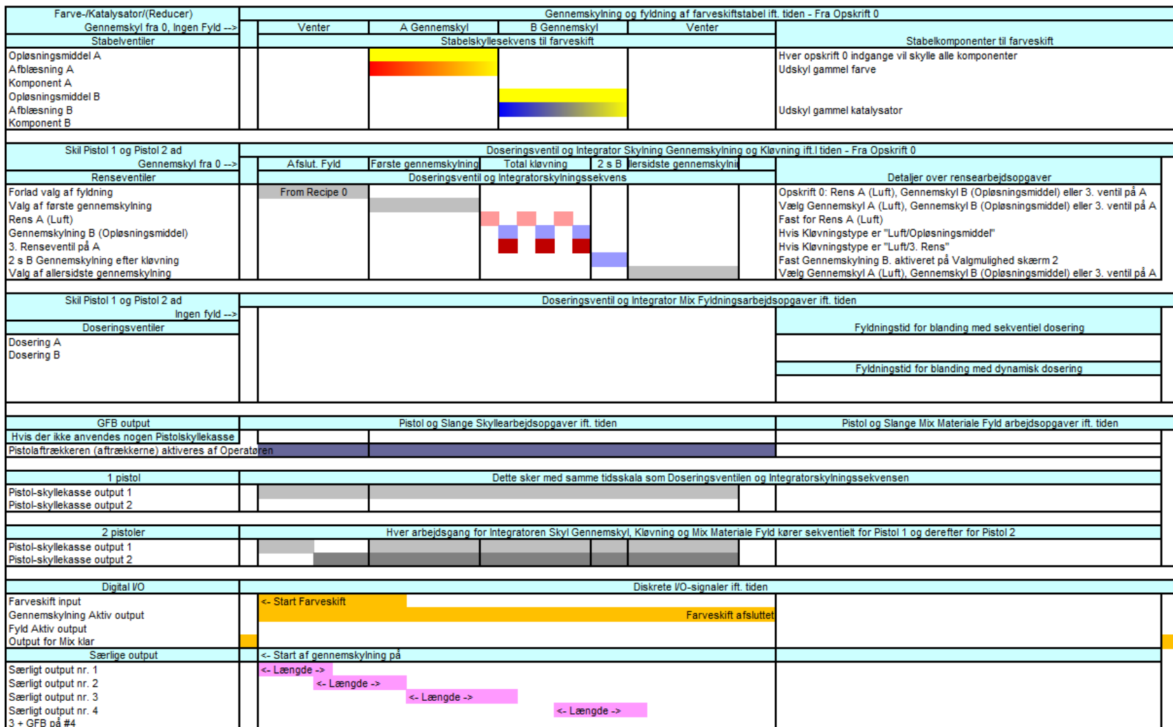
ProMix 2KS Diagram over opskriftgennemskylning nr. 9 0 til 0 Stabelventiler slukket Afbløsnng A aktiveret, 3. Skyleventil aktiveret Forlad fyldning aktiveret
