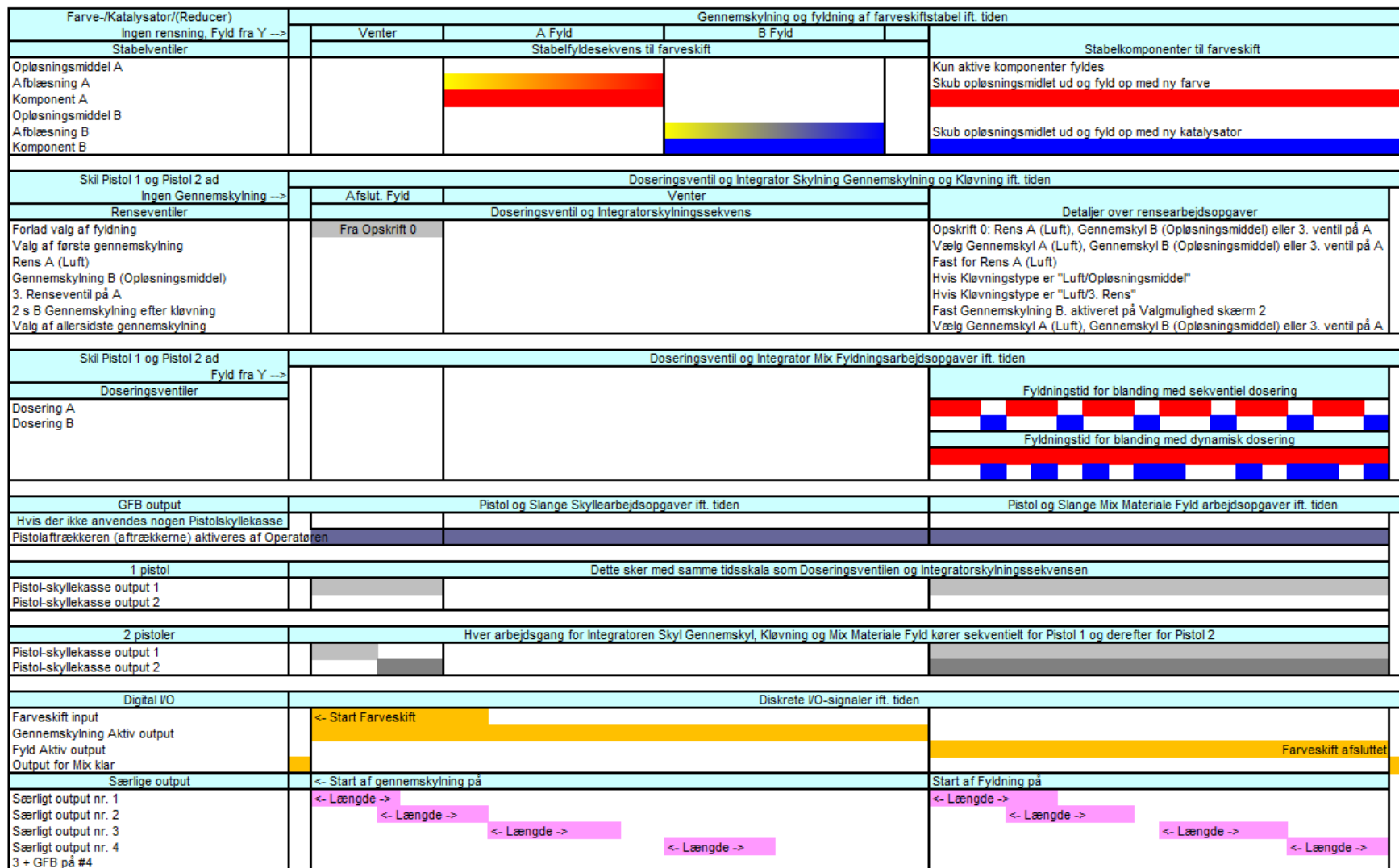
ProMix 2KS Diagram over opskriftfyldning nr. 3 0 til Y Stabelventiler A1, B1 Aflæsning A aktiveret, 3. Skylleventil aktiveret Forlad fyldning aktiveret
