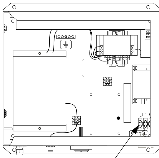
Netzeingang-Anschlussklemmenblock
