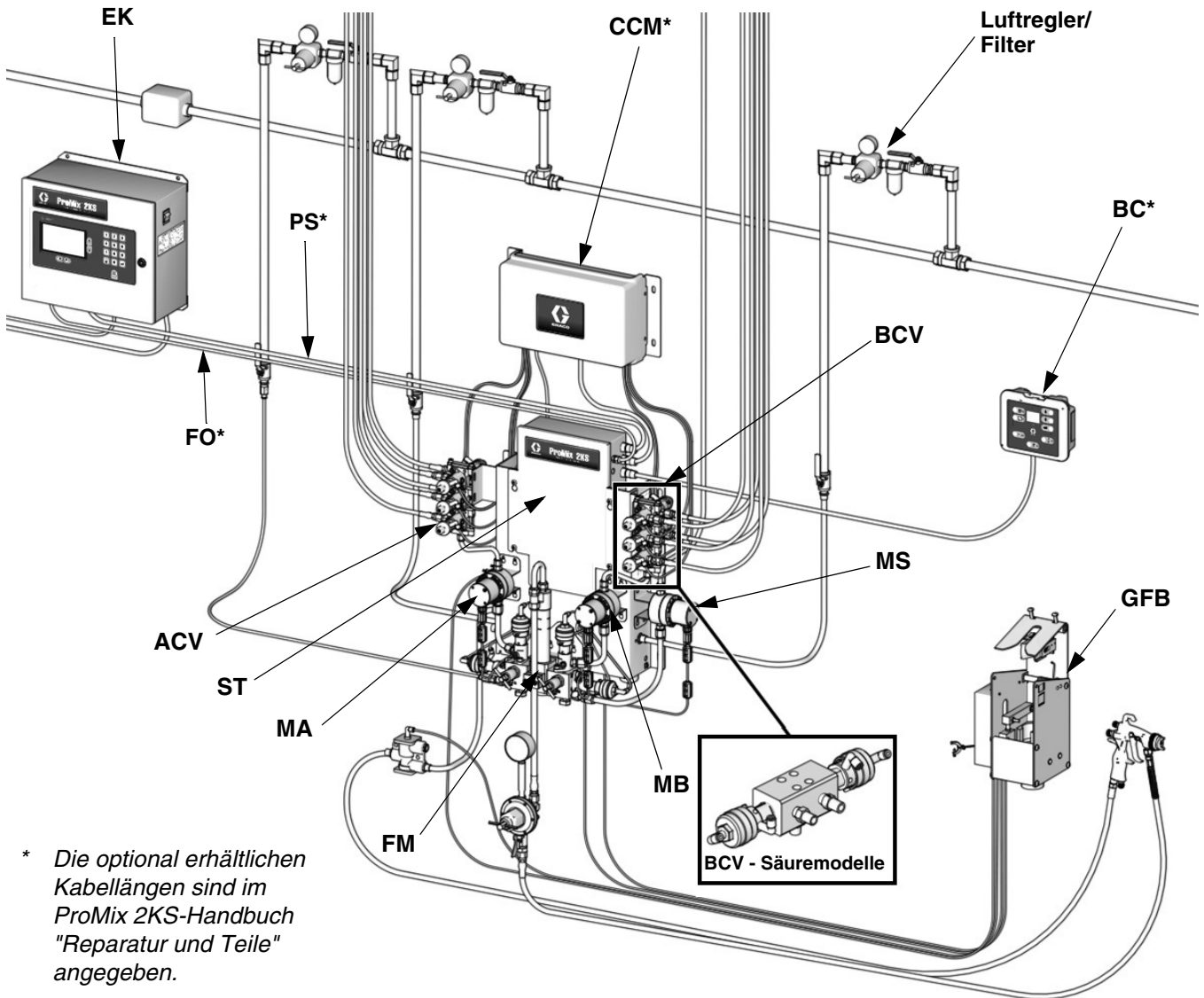
ABB. 2. Manuelles Spritzsystem, dargestellt mit G3000-Volumenzählern, Farb-/Katalysatorwechsel, einem Pistolenspülkasten und zusätzlichem Lösemittel-Volumenzähler
