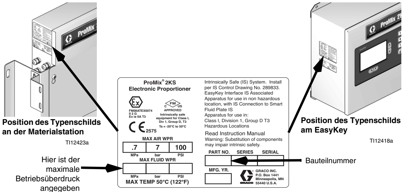
ABB. 1: Typenschild
